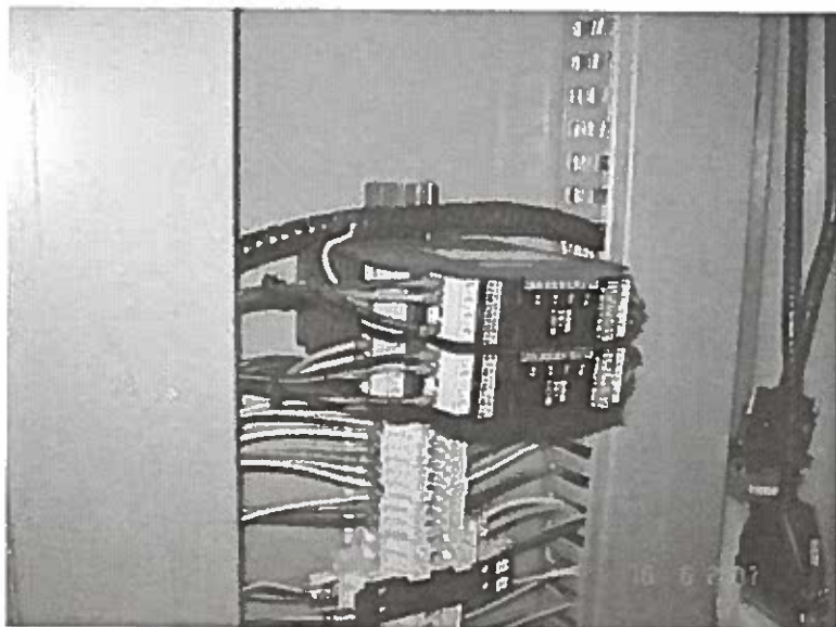
PLC - RELÉ DE SEGURANÇA NÍVEL 4
