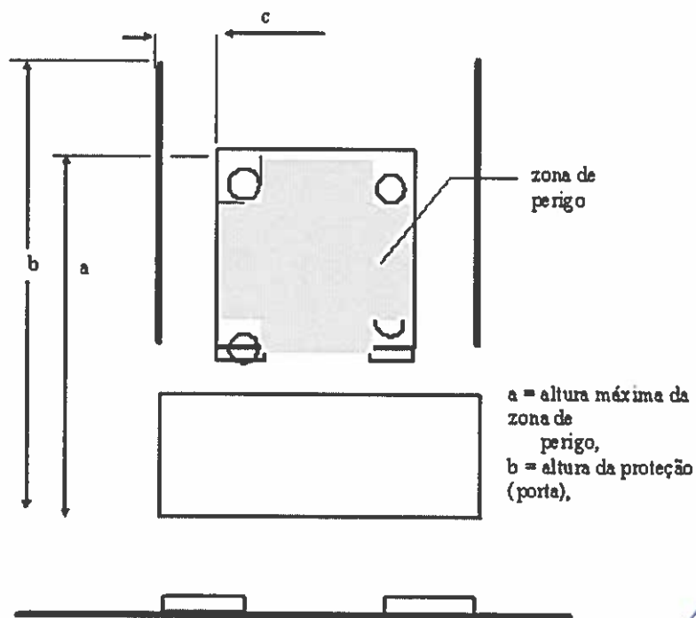
Figura 1 - Proteções sem abas superiores
