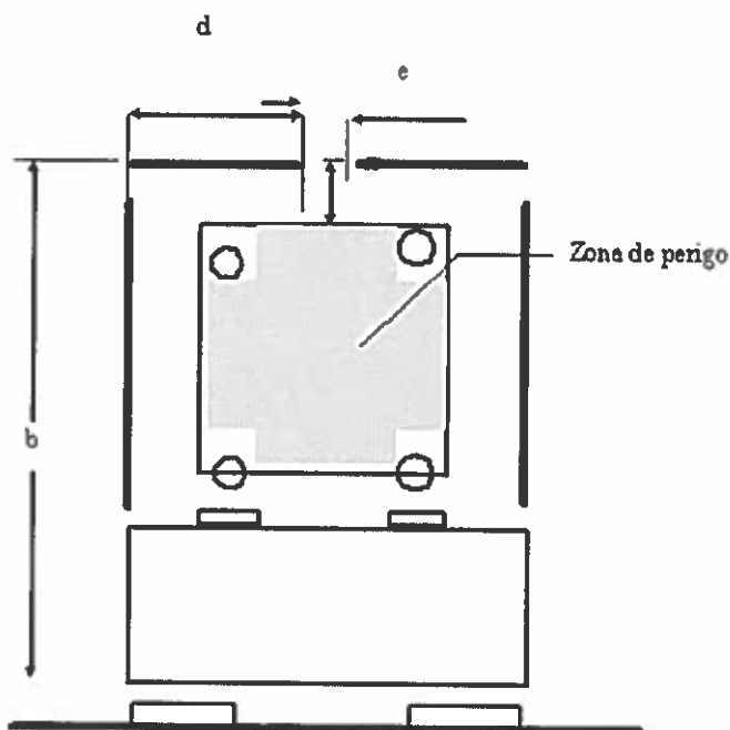
Figura 2 - proteções com abas
