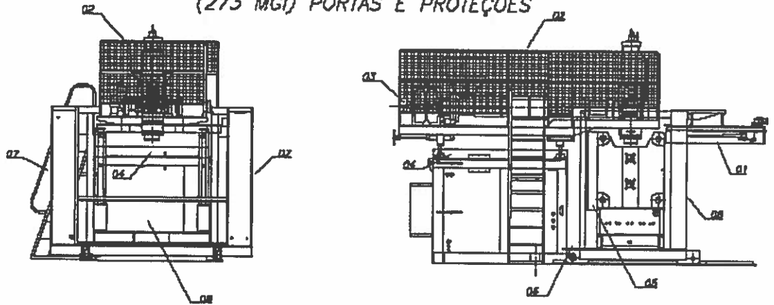
LAY-OUT DIMENCIONAL MAXTEC 30L (273 MGI) PORTAS E PROTEÇÕES
